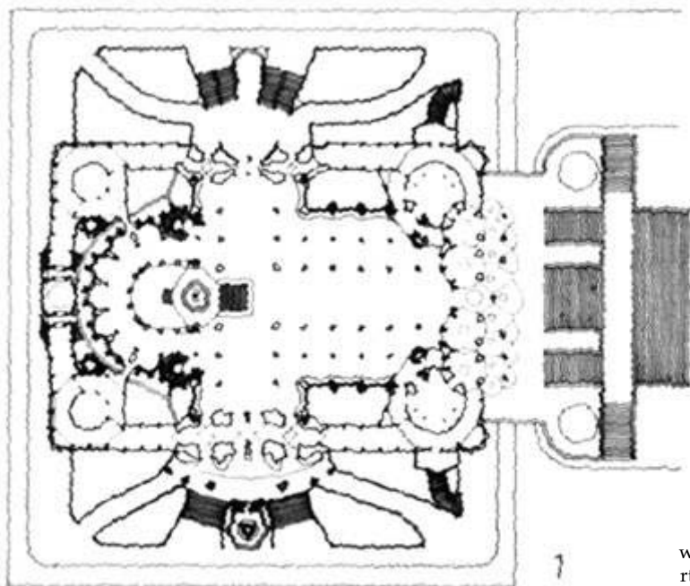
Planta Baixa. Fonte: ZERBST, Rainer. Antoni Gaudí. Taschen, 1985.
